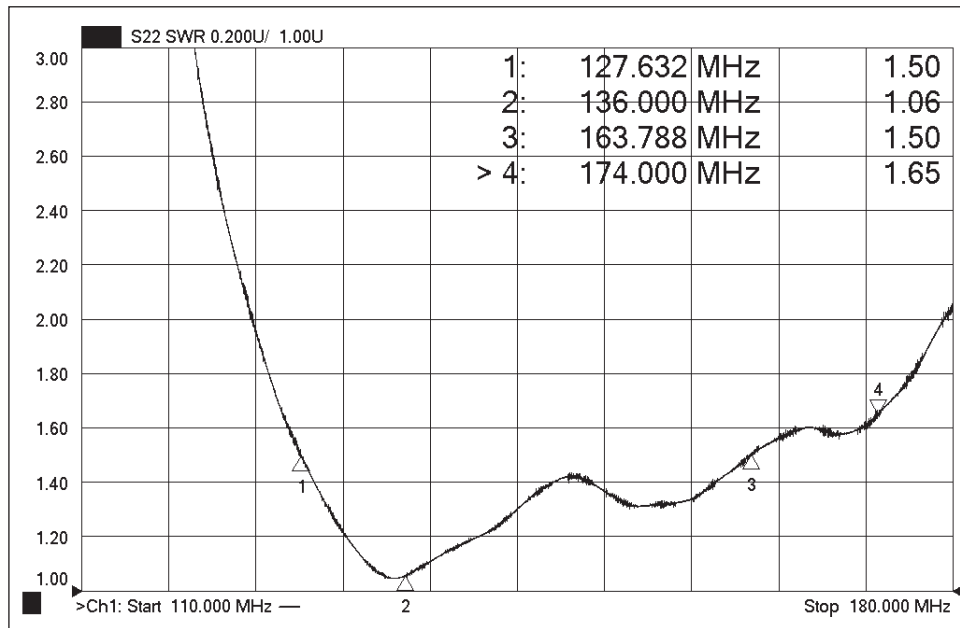
График КСВ
