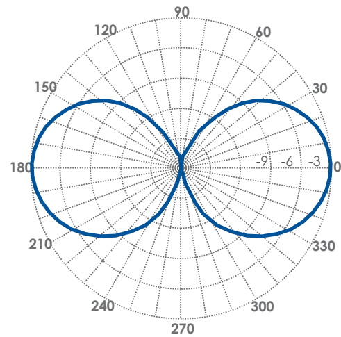
Диаграмма направленности
