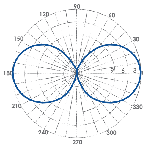
Диаграмма направленности
